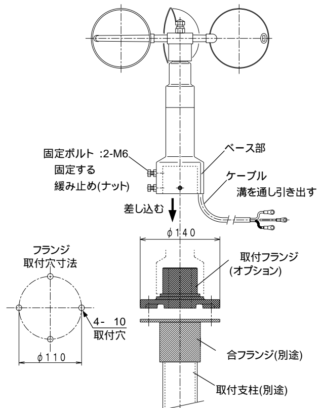
図4.2.2 フランジ式の取付
