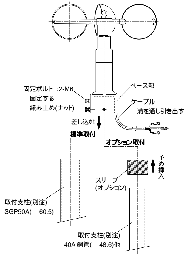
図4.2.1 差込み式の取付
