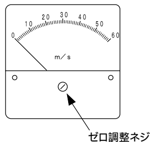
図6.1.2 指示メータ
