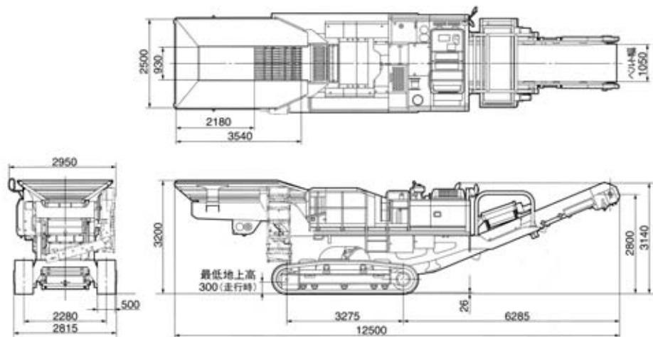
外形図 (単位: mm)
