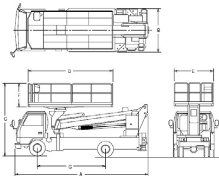
■寸法図(単位:mm)
