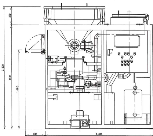
混気ジェットミキサー／AMP-6LT 側面図
