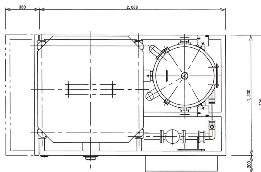
混気ジェットミキサー／AMP-6LT 上面図
