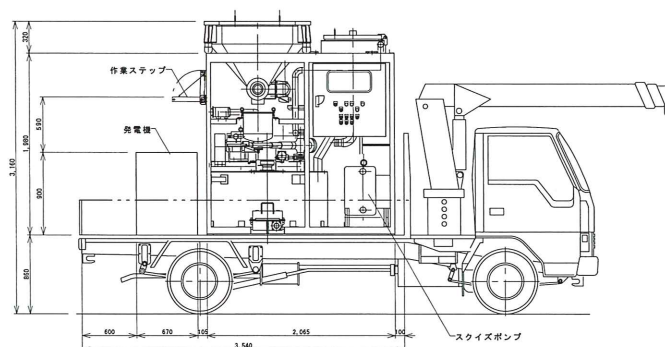
混気ジェットミキサー／AMP-6LT 車載イメージ 側面図
